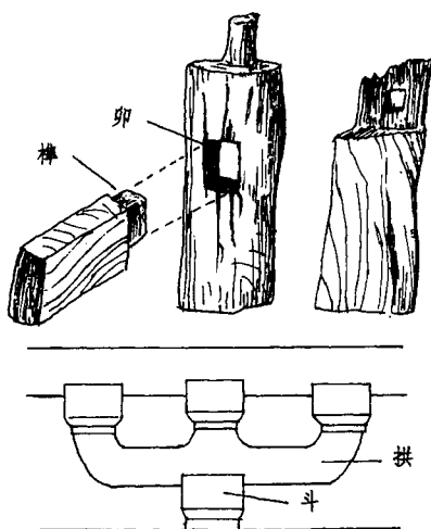
榫卯和斗拱
