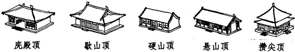
屋顶的五种基本样式
