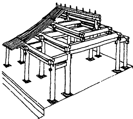
木构架结构
